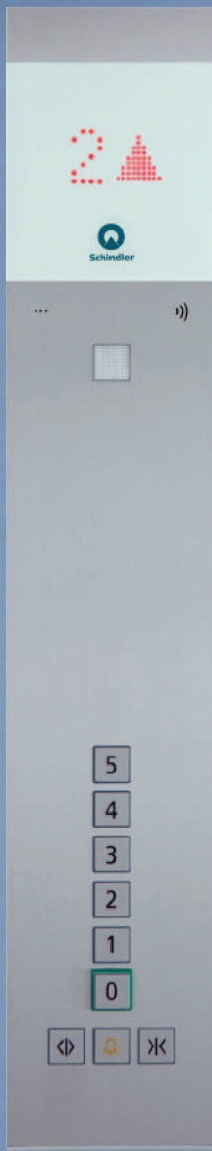
Kabinový ovládací panel (COP), mechanická tlačítka 197 x 1040 mm
